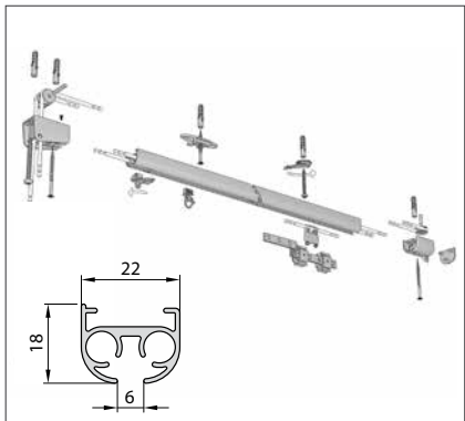
Modell 510 Schnurzugschiene
