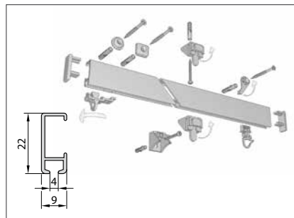
Modell 550 Hochschleuderschiene
