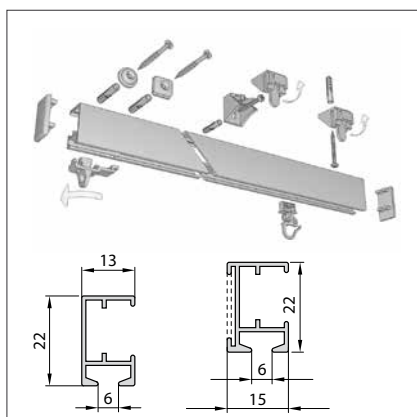
Modell 801,899 Hochschleuderschiene
