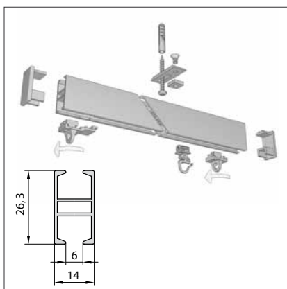
Modell 840 Hochschleuderschiene
