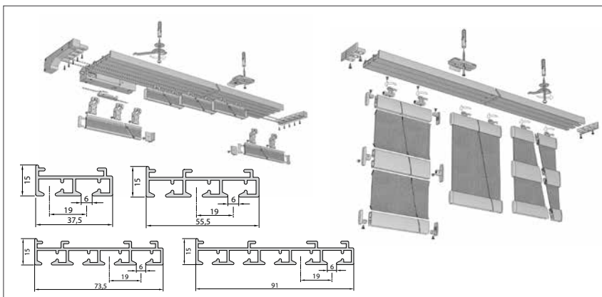
Modell 200-230 Flächenvorhangschiene
