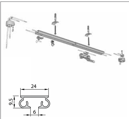
Modell 505 Schnurzugschiene
