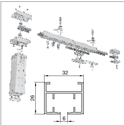
Modell 670 Elektrosciene
