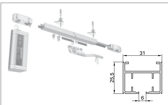
Modell 620 Elektrosciene
