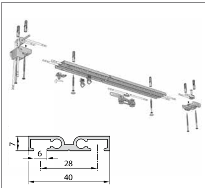
Modell 815 Schnurzugschiene
