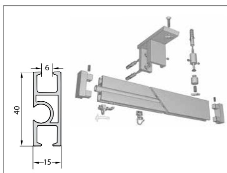
Modell 700 Dekorschiene
