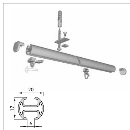
Modell 440 Rundrohrschleuderschiene
