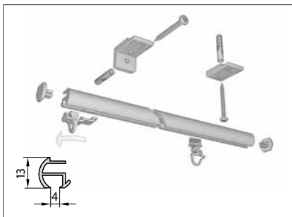
Modell 545 Schleuderschiene
