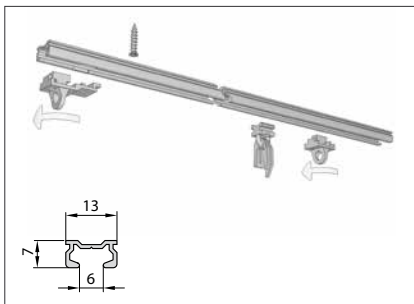
Modell 810 Flachschleuderschiene
