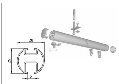
Modell 865 Rundrohrschleuderschiene
