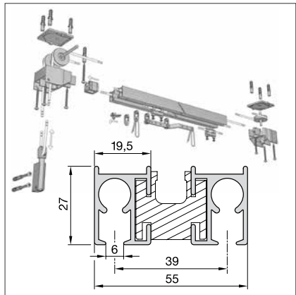
Modell 886 Seilzugschiene
