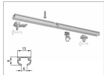
Modell 800 Flachschleuderschiene
