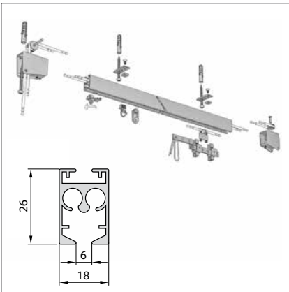
Modell 820 Schnurzugschiene
