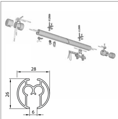
Modell 845 Schnurzugschiene
