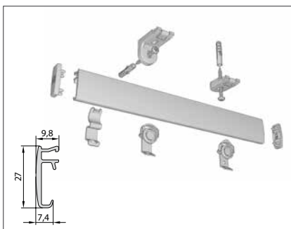
Modell 750 Objektschleuderschiene
